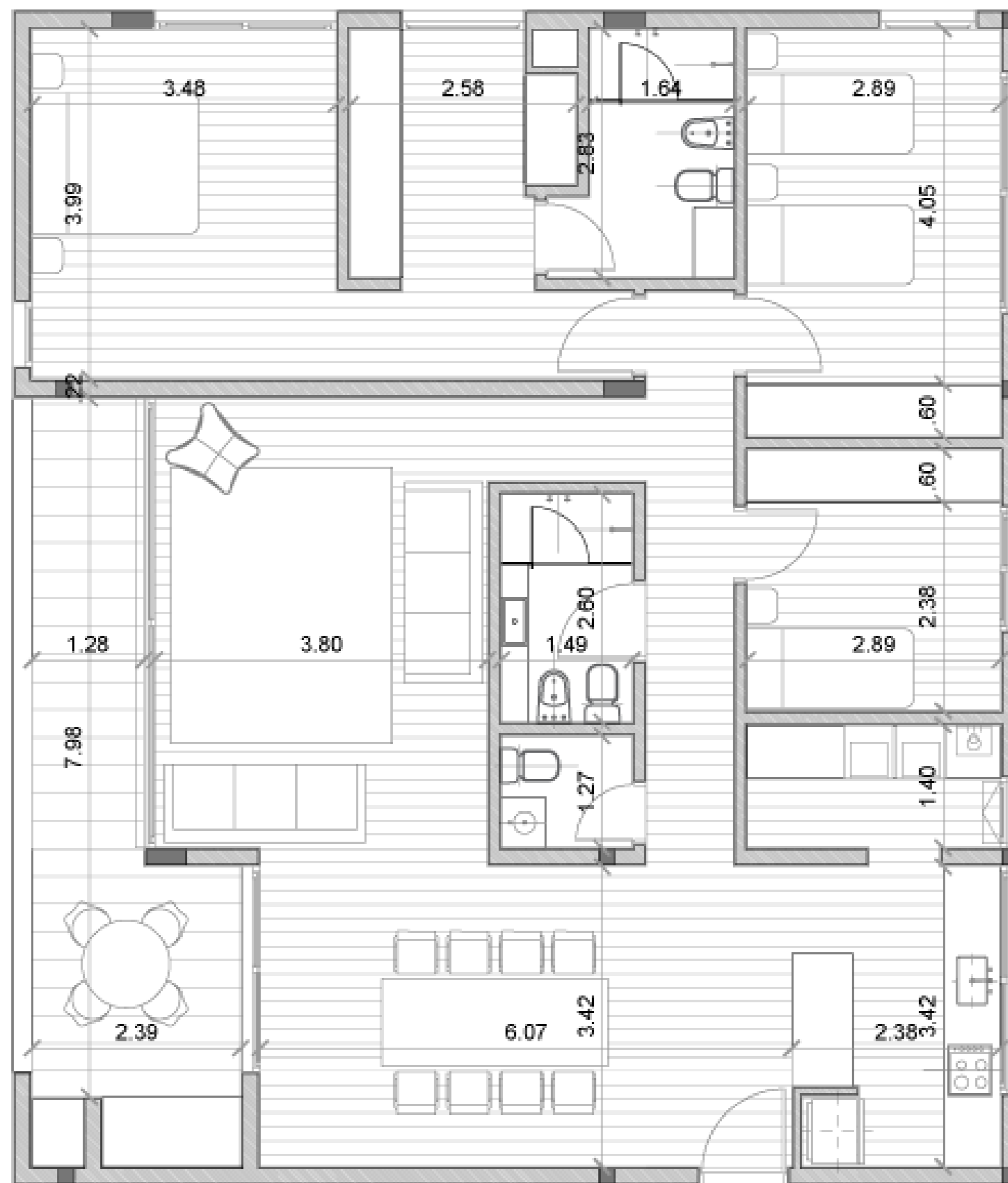
PROTOTIPO 2 | Esc. 1:100
