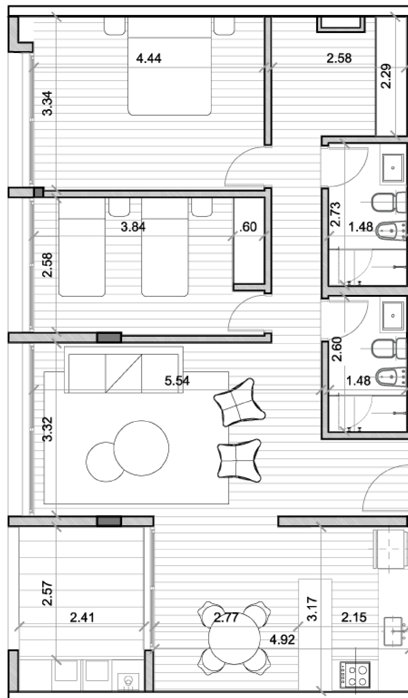
PROTOTIPO 3 | Esc. 1:100
