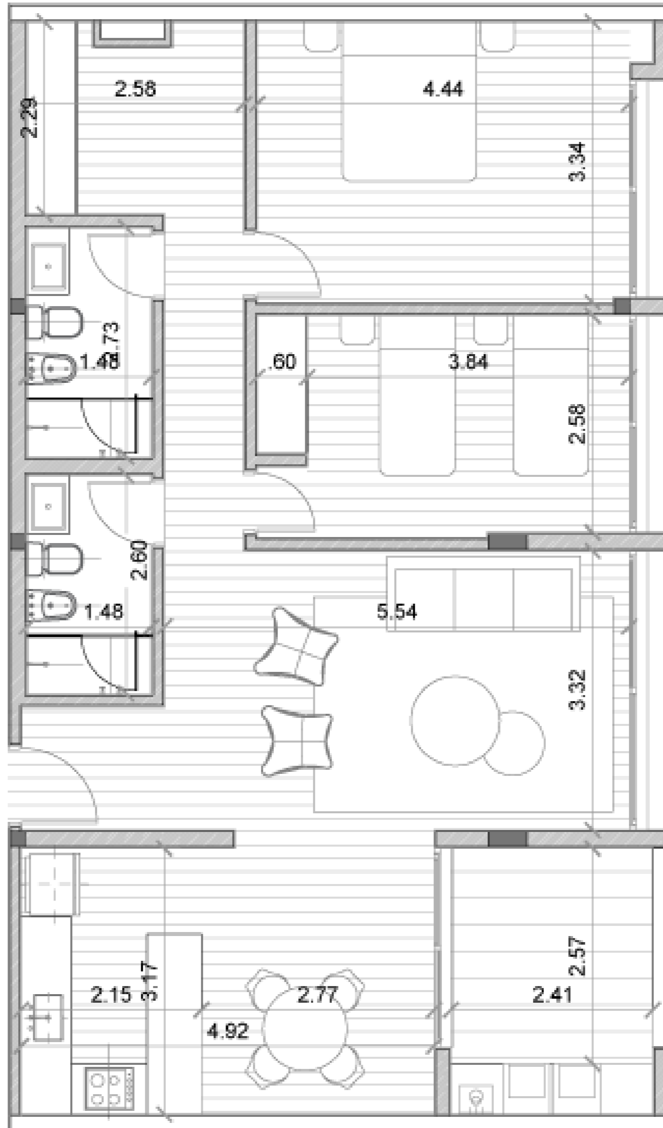
PROTOTIPO 3 | Esc. 1:100
