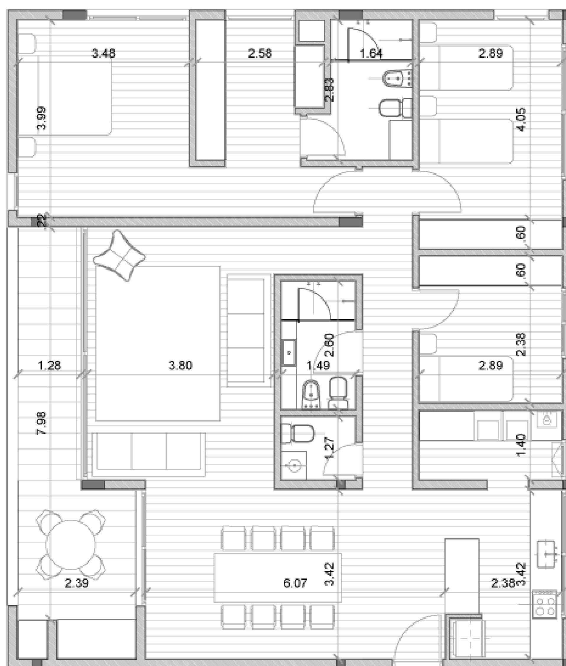
PROTOTIPO 2 | Esc. 1:100
